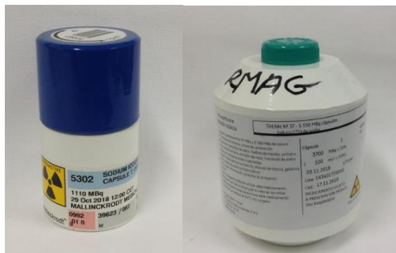
Figura 34. Cápsulas de 1110 MBq y 5550 MBq de ^{131}\text{I} en envases con medidas de radioproteccion.
